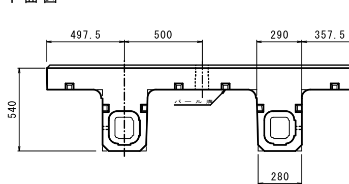
下面図
