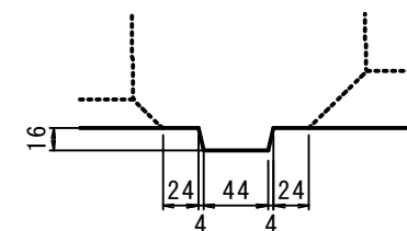
A 詳細図
