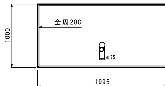
正面図
