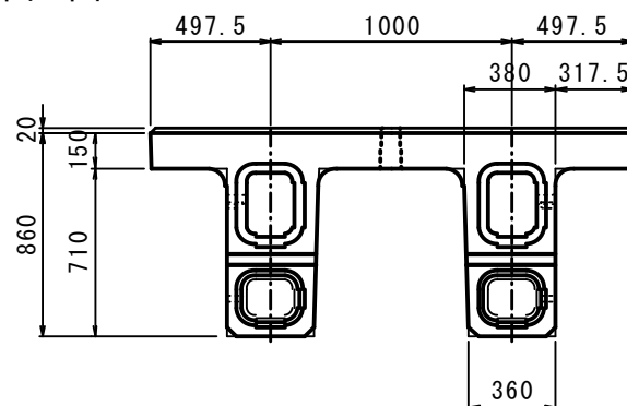
上面図
