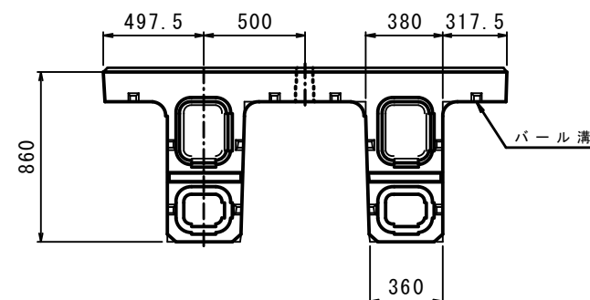
下面図
