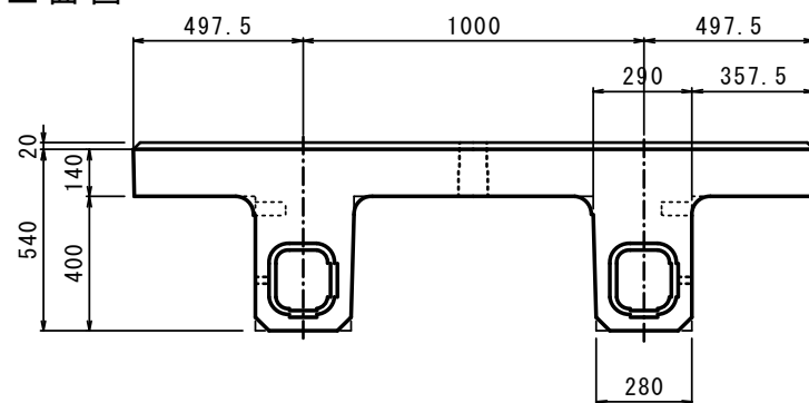
上面図
