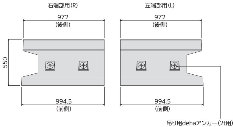
上面図
